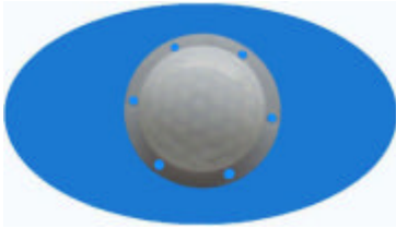
型号：8341 焦距：15 角度：120° 距离：10m 尺寸：外径 44.6 内径 35.00
