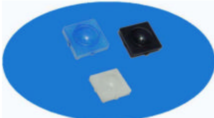
型号：8109 直径：24mm 焦距：9mm 厚度：0.7mm 角度：100°
