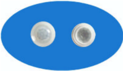
型号：7709-3 焦距：11.0 角度：120° 距离：8m 尺寸：外径 17.8 内径 12
