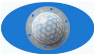
型号：8320-6 焦距：17.5 角度：120° 距离：14m 尺寸：32 外径 45.3 高 11.00
