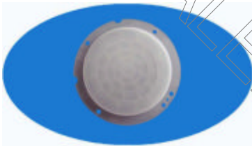
型号：8102-1 焦距：15 角度：120° 距离：8m 尺寸：内径 36 外径 45
